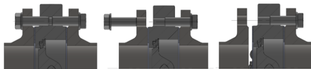
Obr. 10: Demontáž příruby za klapkou
