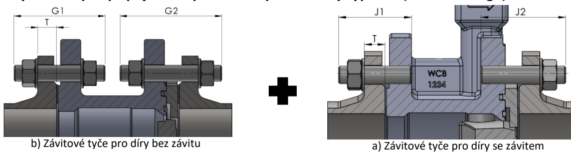
Obr. 13: Rozměry spojovacího materiálu pro klapky s tělesy typu DF (Double Flange)
