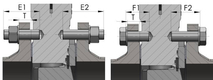
Obr. 12: Rozměry spojovacího materiálu pro klapky DN450-600 s tělesy typu B a T
