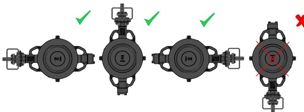
Obr. 6: Doporučené polohy klapky při montáži do potrubí
