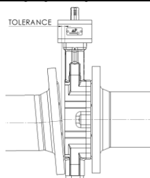
Obr. 4: Rovnoběžnost přírub
